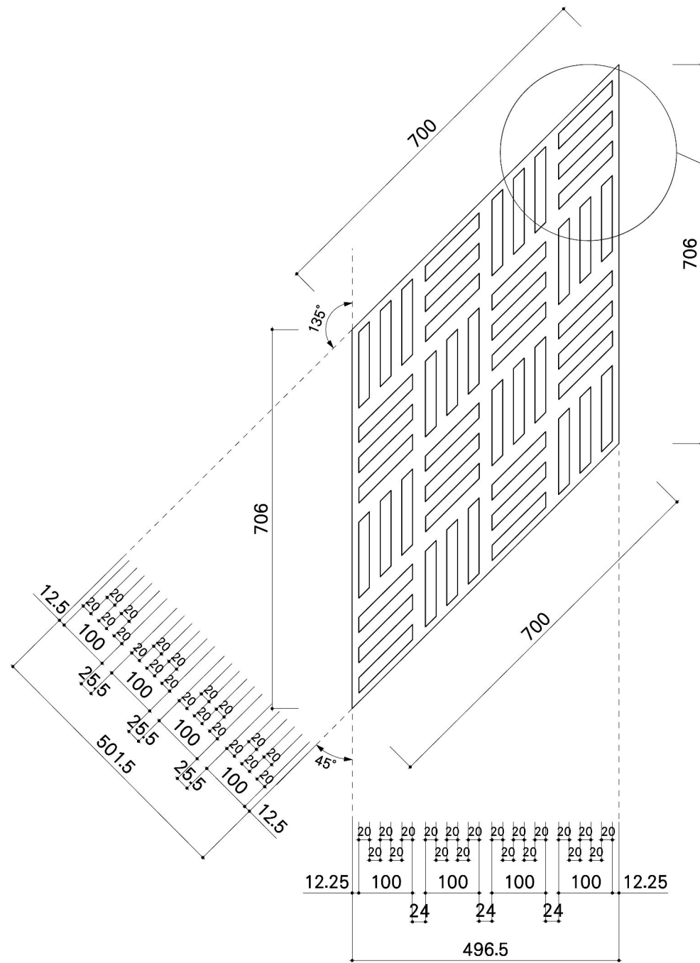
製品マット図 S1/10
