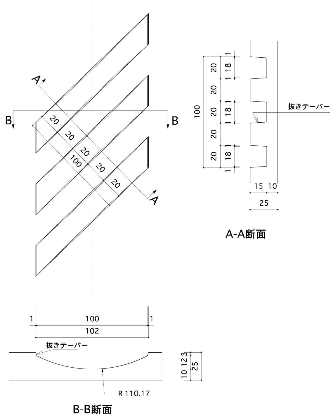
意匠部拡大詳細図 S=1/2
